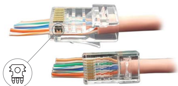
PLEZ-8P8C-U-C6
